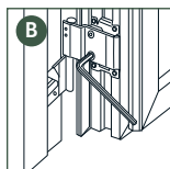
5 mm unbraconøgle
