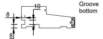
Groove bottom
